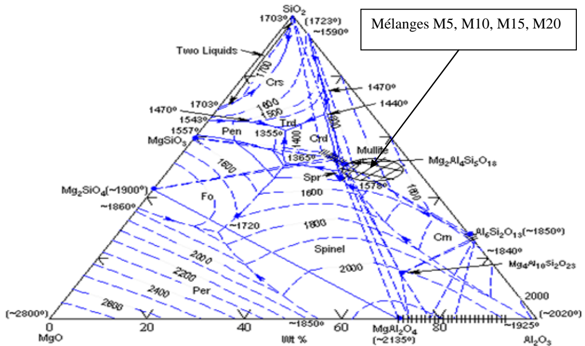
Figure 4.8 Diagramme ternaire des phases du système MgO-Al 2 O 3 -SiO 2 (MAS) d'après [81].
