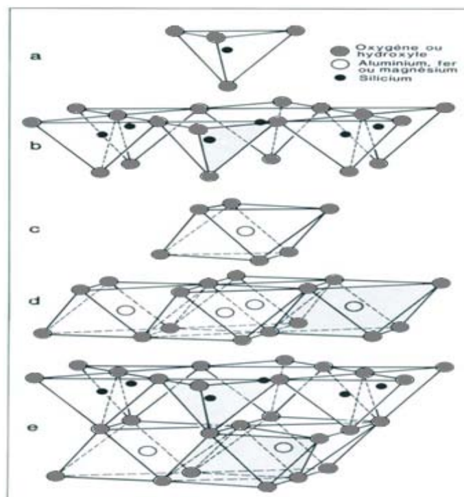
Figure 2.1 Structure de la kaolinite, a) tétraèdre de silice, b) couche de tétraèdres de silice, c) octaèdre d'alumine, d) couche d'octaèdres d'alumine, e) feuillet de kaolinite.
