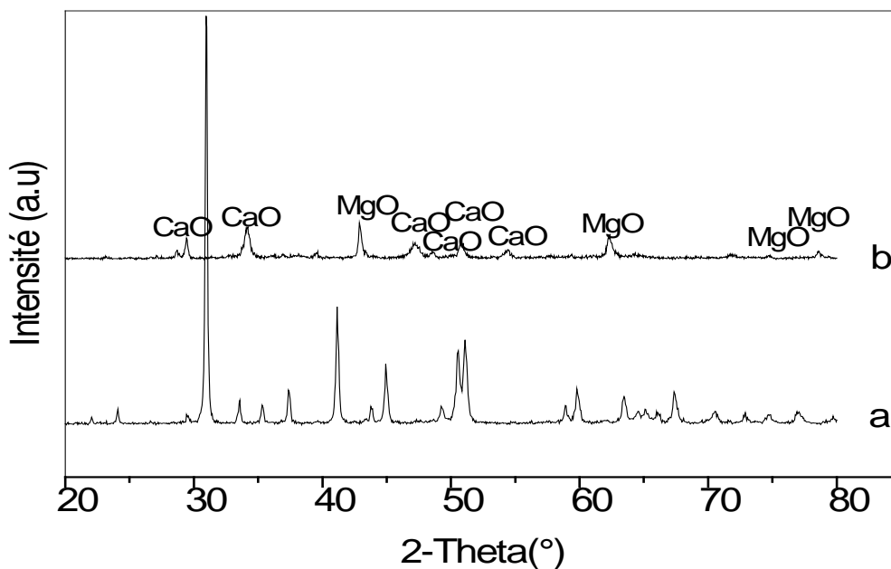
Figure 5.3 Diffraction aux rayons X de la dolomie, a) Etat naturel, b) Calcinée à 900°C, pendant 2 heures.
