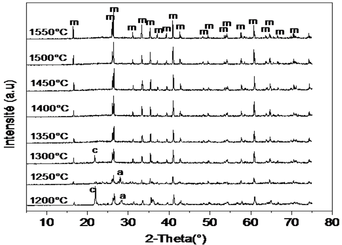
Figure 5.7 DRX du mélange M5 fritté entre 1200°C-1550°C, pendant 2h, (a : Anorthite, c : Cristobalite, m : Mullite).
