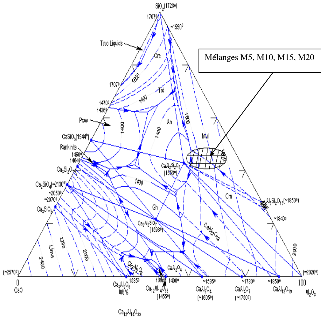
Figure 4.7 Diagramme ternaire des phases du système CaO- Al 2 O 3 -SiO 2 (CAS) d'après [80].
