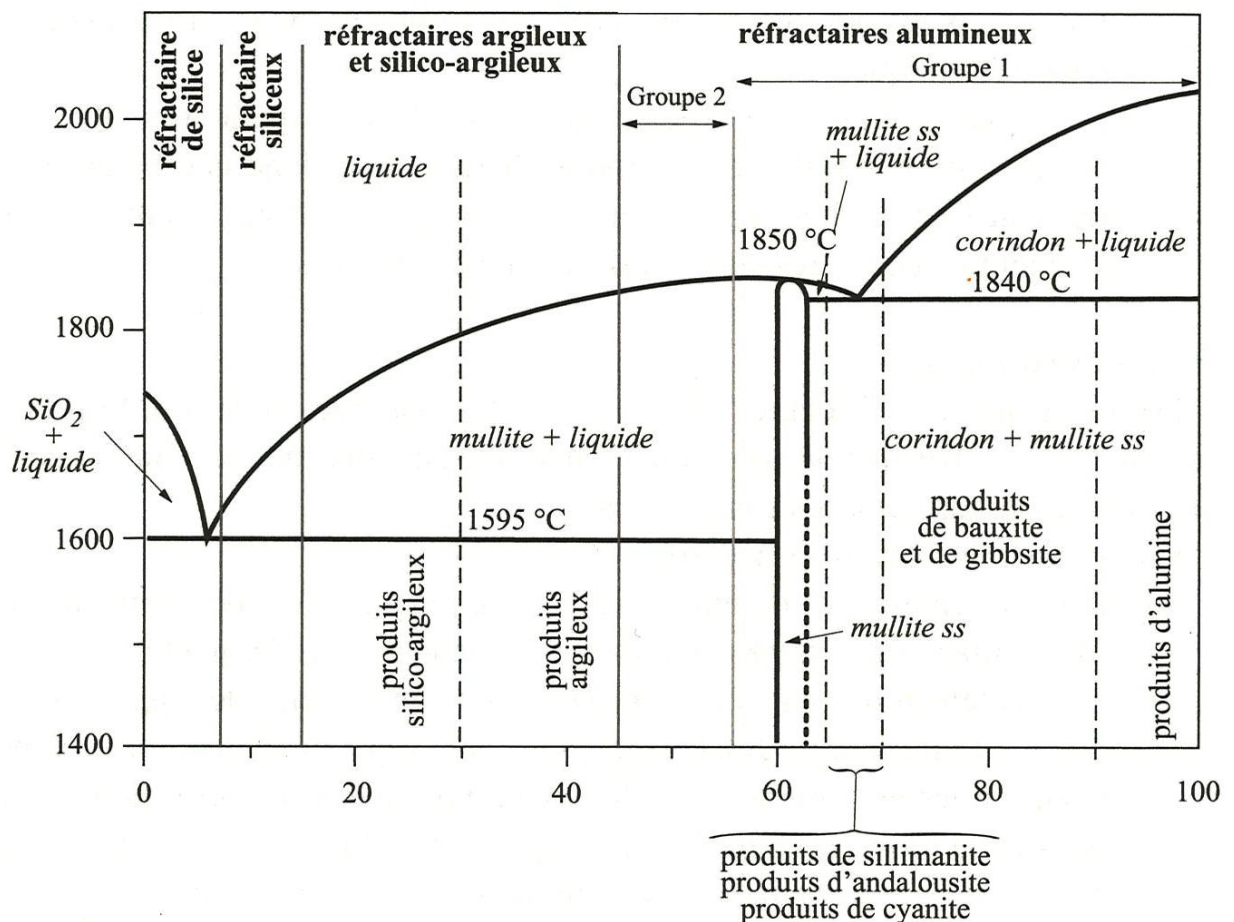
Figure 1.1 Diagramme de phases Al_2O_3 - SiO_2 des réfractaires alumino-silicatés [3].
