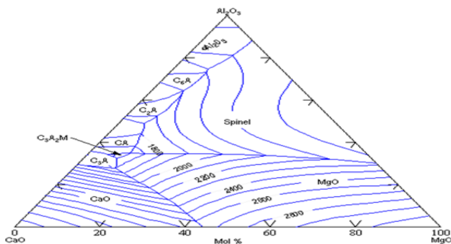
Figure 4.9 Diagramme ternaire des phases du système MgO-Al 2 O 3 -CaO (MAC) d'après [82].
